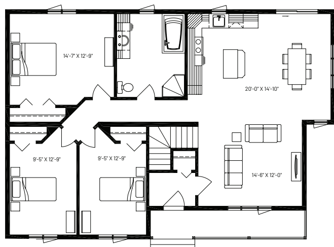
REZ-DE-CHAUSSÉE
