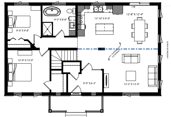
REZ-DE-CHAUSSÉE
