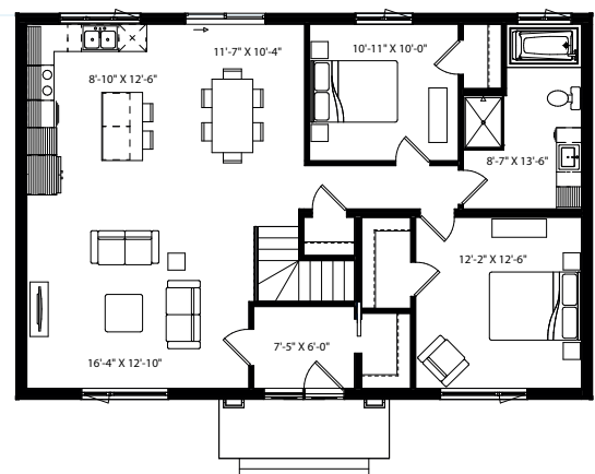
REZ-DE-CHAUSSÉE
