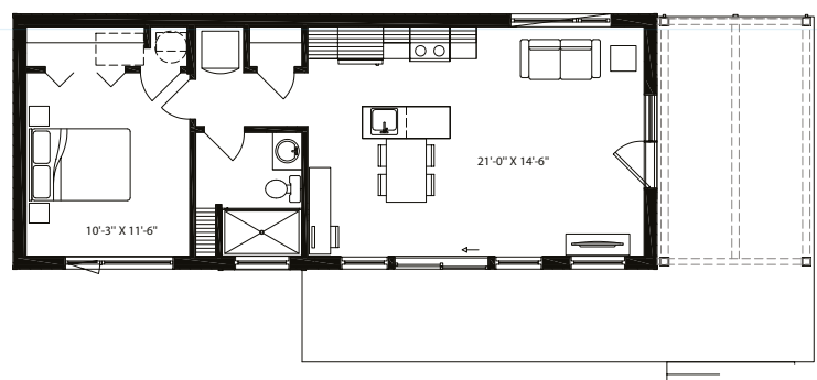
REZ-DE-CHAUSSÉE
