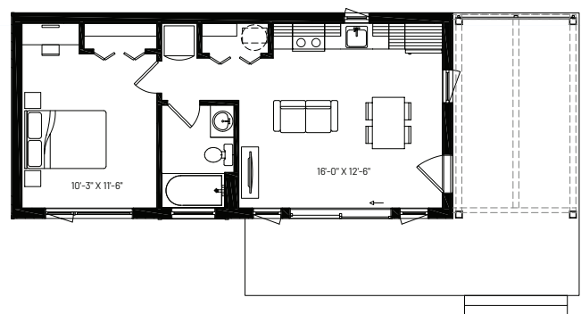
REZ-DE-CHAUSSÉE
