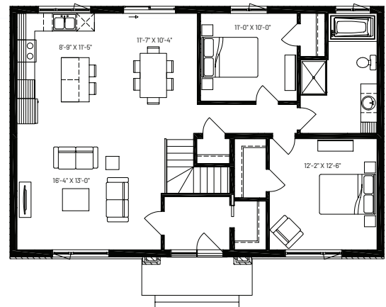
REZ-DE-CHAUSSÉE
