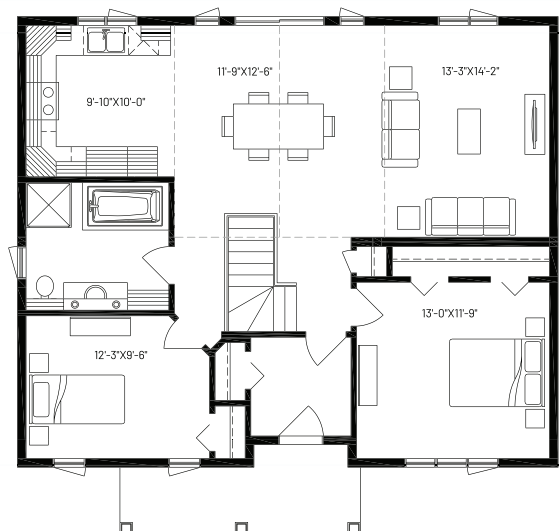
REZ-DE-CHAUSSÉE
