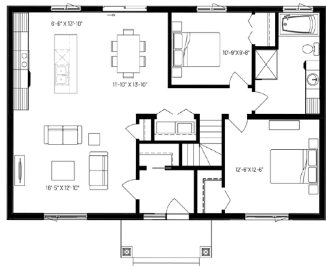
REZ-DE-CHAUSSÉE
