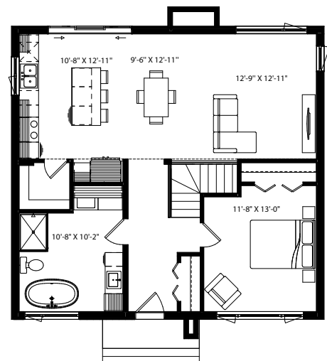
REZ-DE-CHAUSSÉE
