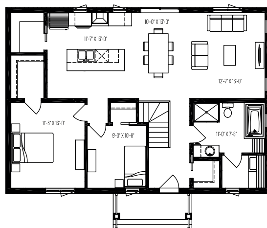
REZ-DE-CHAUSSÉE
