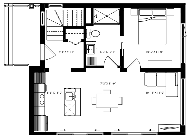
REZ-DE-CHAUSSÉE
